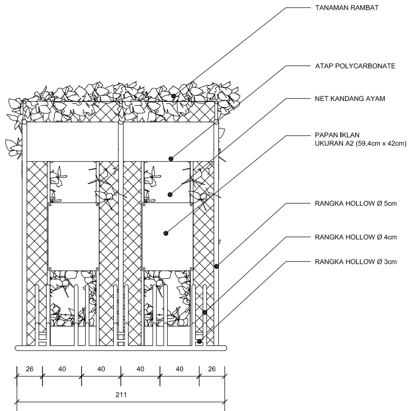
TAMPAK DEPAN
